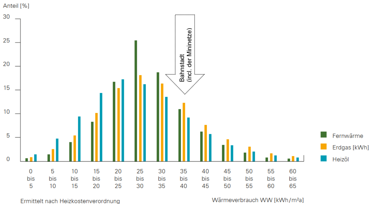
Abbildung 11: Häufigkeitsverteilung des flächenbezogenen Wärmeenergieverbrauchs für die Trinkwassererwärmung im Bundesdurchschnitt, Bezug auf Wohnfläche (aus [Techem 2019], nicht witterungsbereinigt)
