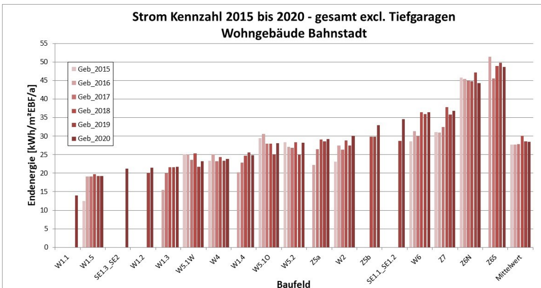
Abbildung 14: Strom gesamt excl. Tiefgaragen
