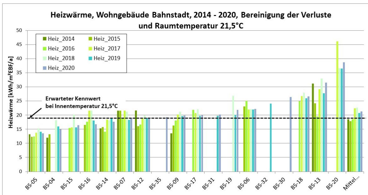
Abbildung 5: Heizwärme der Wohnbaufelder, Verluste witterungsbereinigt, Messabweichung \pm 4 kWh/(m 2 a)
