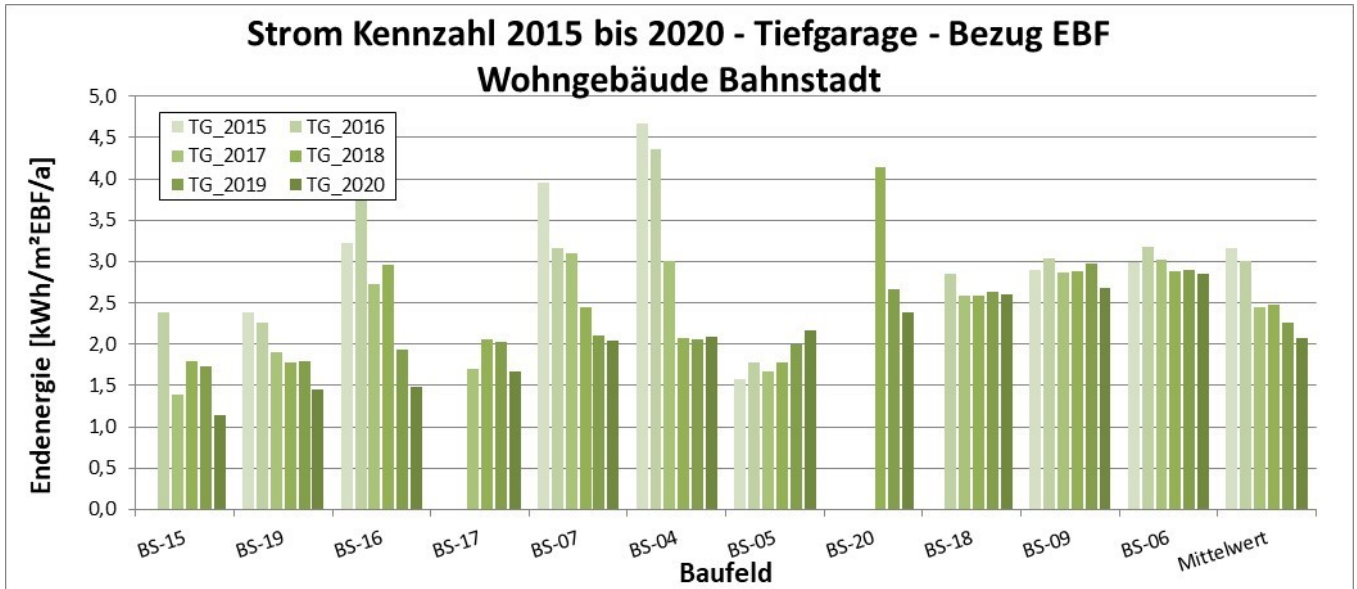
Abbildung 19: Strom Tiefgarage, Bezug EBF
