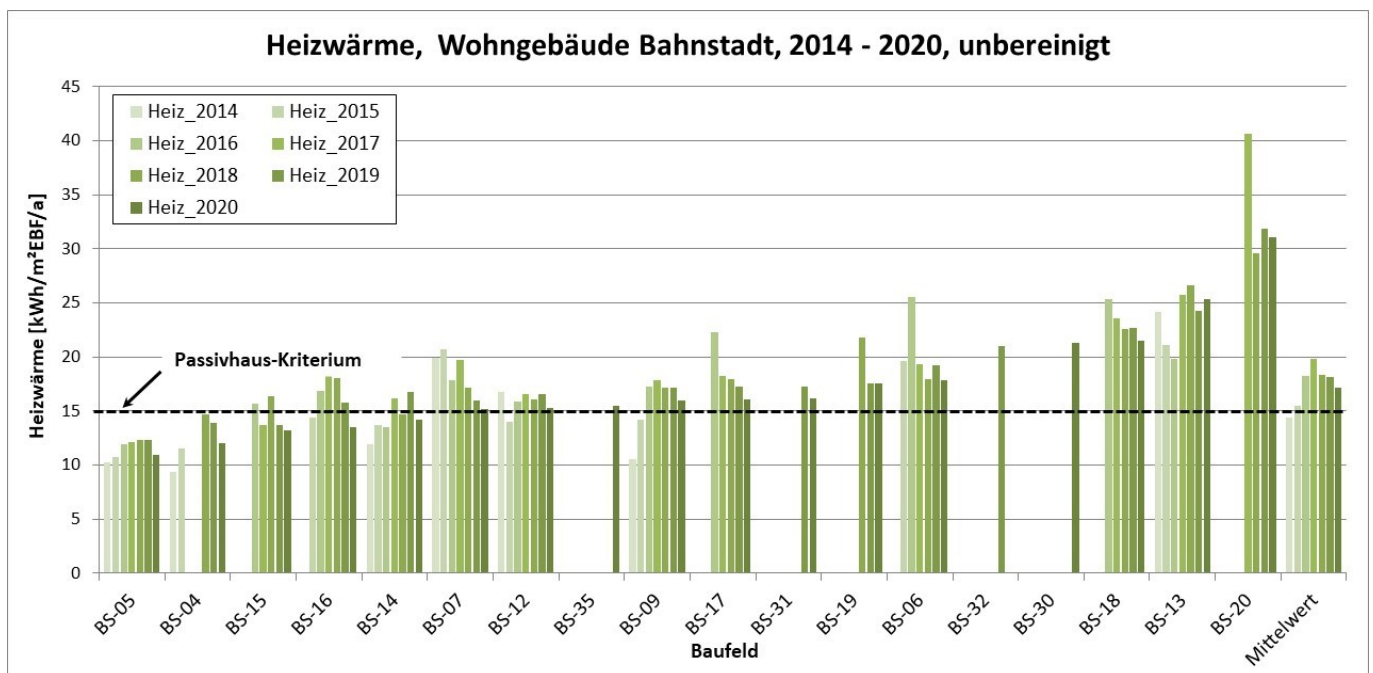
Abbildung 3: Heizwärme der Wohnbaufelder, unbereinigt, Messabweichung im Bereich \pm 4 \text{ kWh}/(\text{m}^2\text{a})
