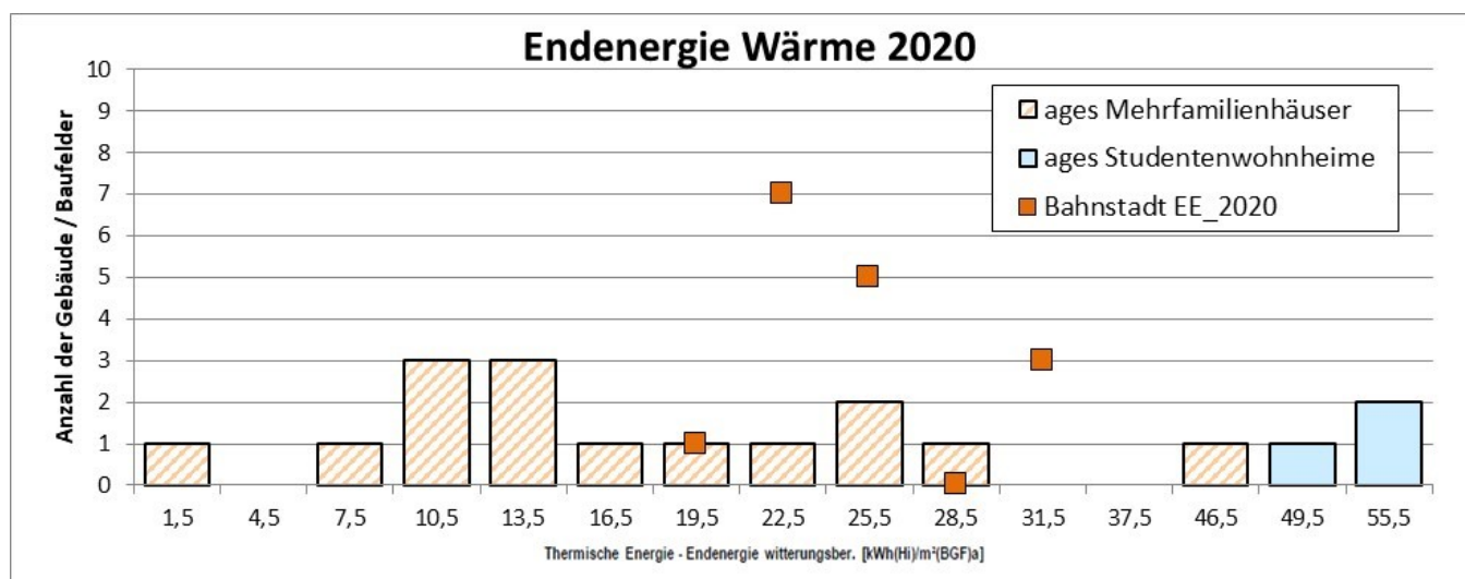
Abbildung 8: Wärmeverbrauch – Häufigkeitsverteilung (in Anlehnung an [ages 2015], Grafik 22)
