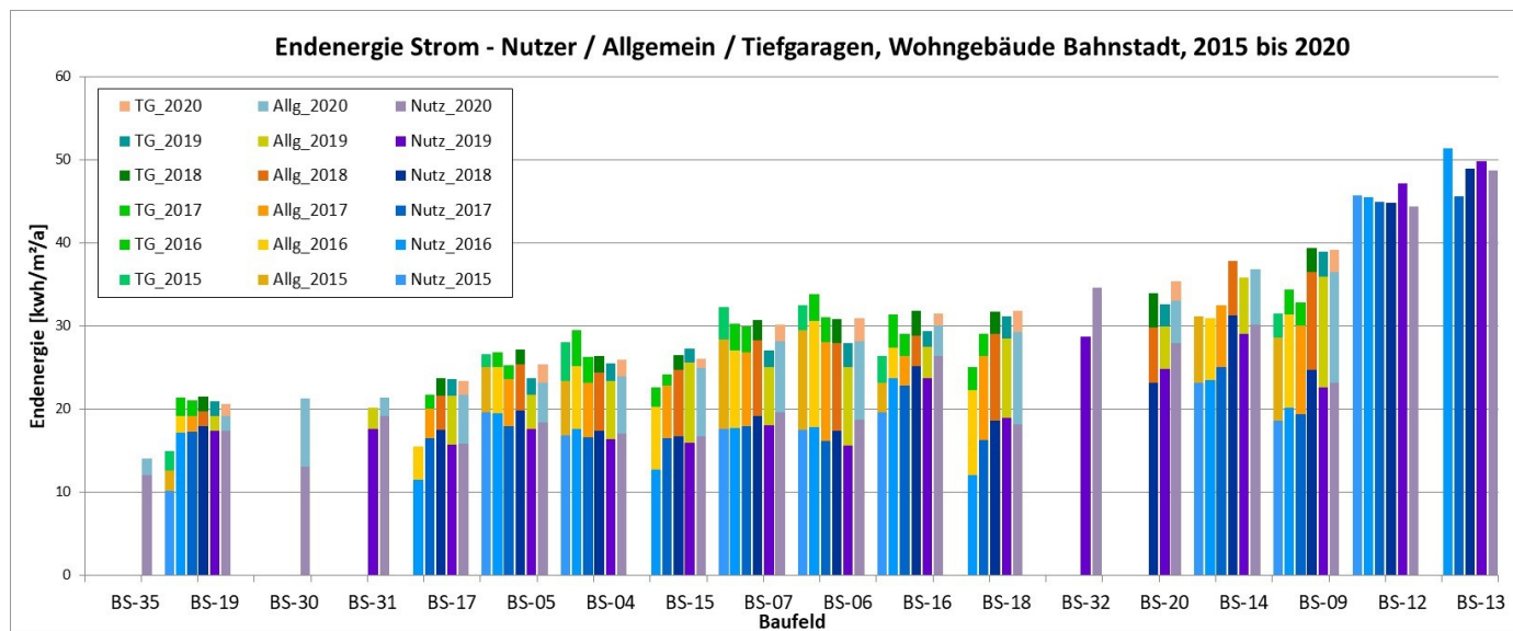
Abbildung 15: Strom gesamt - aufgetrennt
