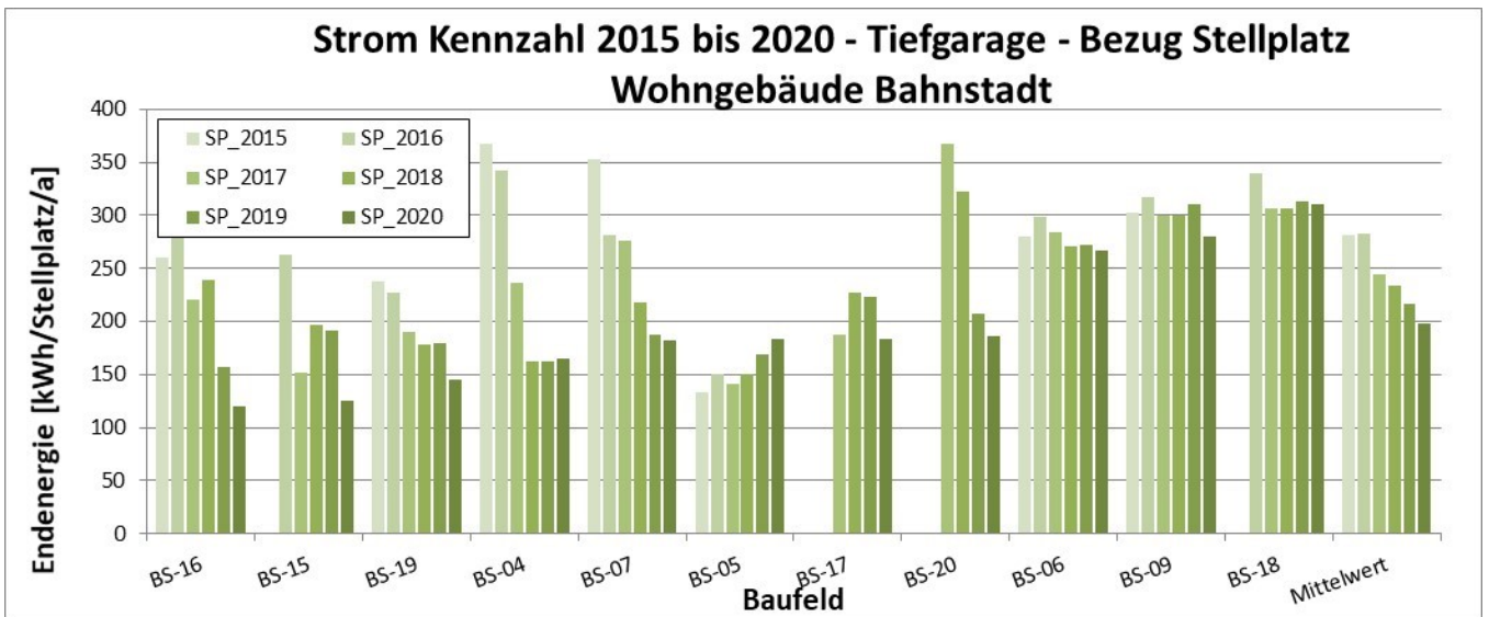
Abbildung 20: Strom Tiefgarage, Bezug Stellplatz
