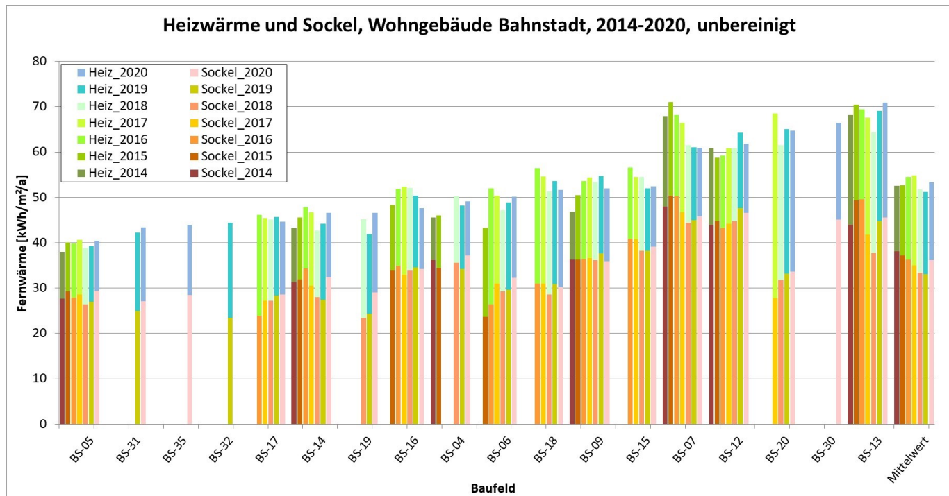
Abbildung 2: Heizwärme und Sockel
