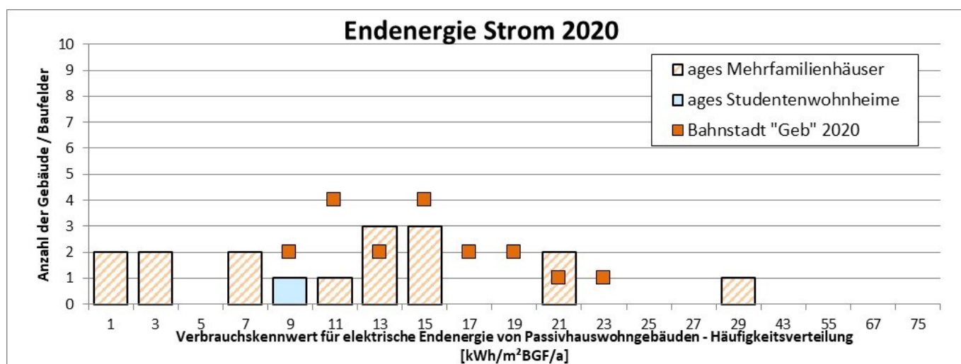
Abbildung 21: Stromverbrauch – Häufigkeitsverteilung (in Anlehnung an [ages 2015], Grafik 20)
