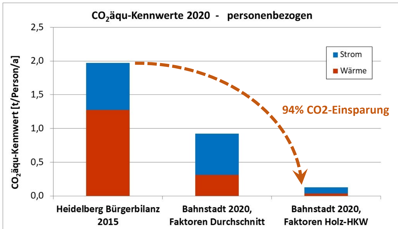
Abbildung 23: CO 2 -Emissionen, Kennwerte pro Person
