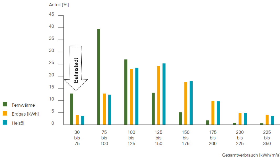
Abbildung 10: Häufigkeitsverteilung des spezifischen Gesamtverbrauchs in verbundenen Anlagen im Bundesdurchschnitt, Bezug auf Wohnfläche (aus [Techem 2019], nicht witterungsbereinigt)
