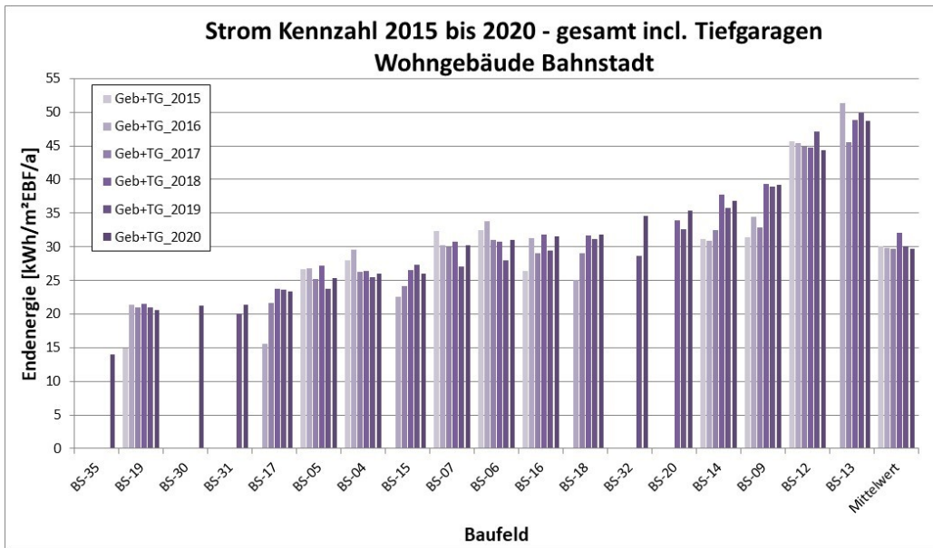
Abbildung 13: Strom gesamt incl. Tiefgaragen
