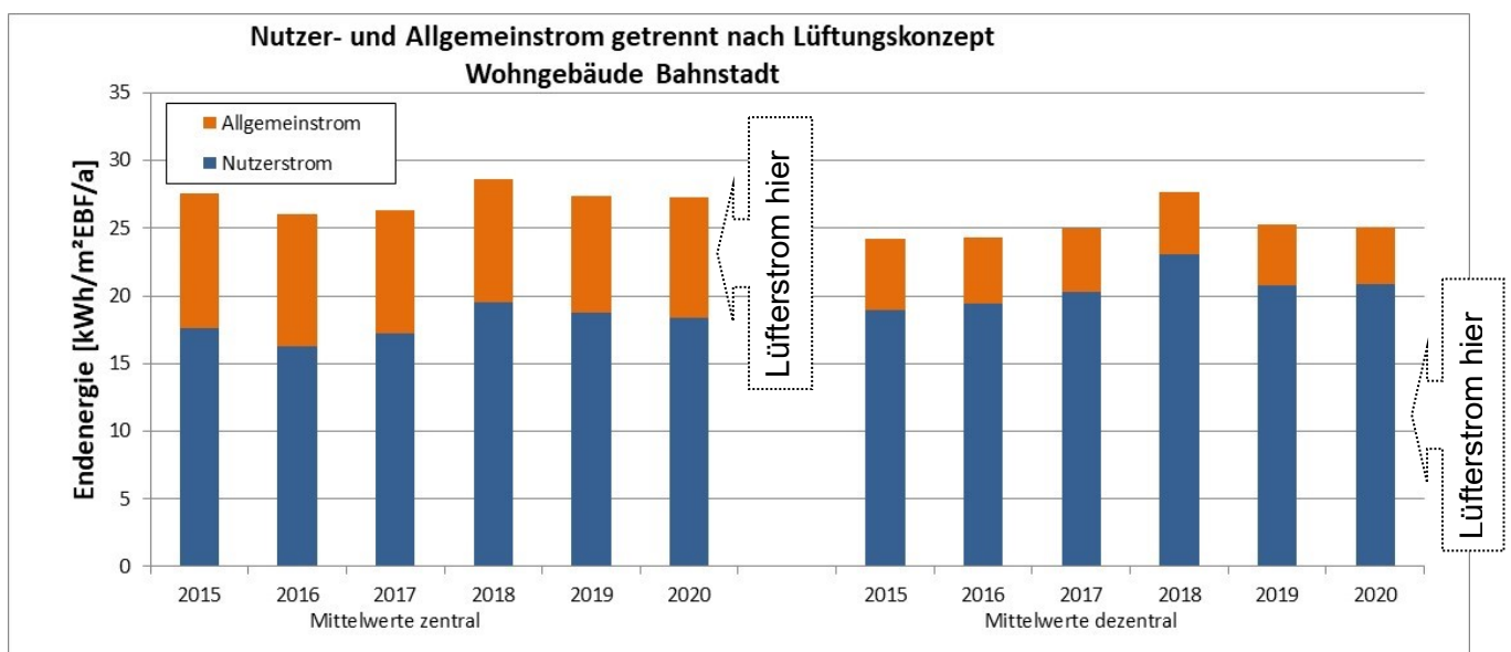
Abbildung 17: Mittelwerte der Baufelder mit zentralem / dezentralen Lüftungskonzept
