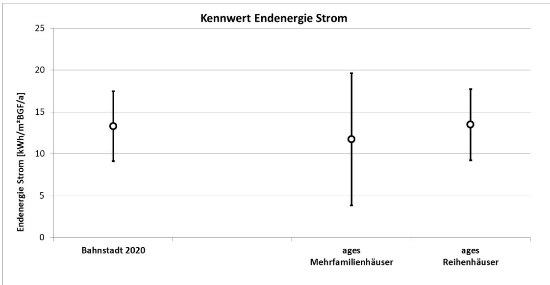
Abbildung 22: Kennwert Endenergie Strom – Mittelwert und Standardabweichung
