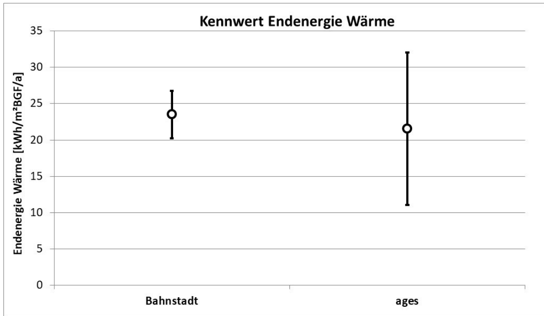
Abbildung 9: Kennwert Endenergie Wärme – Mittelwert und Standardabweichung
